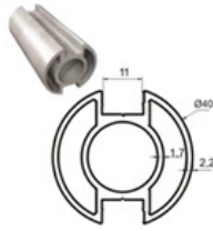
ΚΟΛΩΝΑ ΒΑΡΕΩΣ ΤΥΠΟΥ HEAVY COLUMN TE 3004
