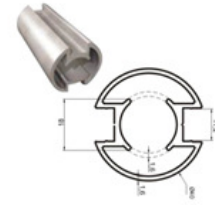
ΚΟΛΩΝΑ ΕΛΑΦΡΟΥ ΤΥΠΟΥ LIGHT COLUMN TE 3004B
